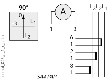
Commutateur d'ampèremètre
