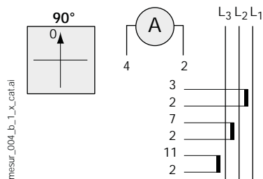
Commutateur d'ampèremètre
