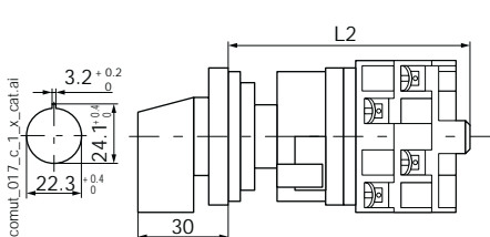
Fixation centrale
