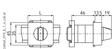
Commutateur
