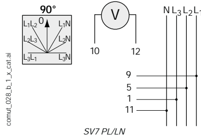
Commutateur de voltmètre - 7 positions :
