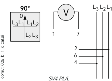
Commutateur de voltmètre
