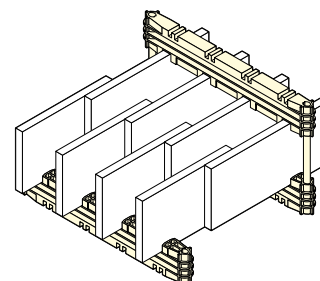
Монтаж одной или двух шин на полюс
