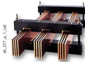
Шинодержатели с фиксированным межфазным расстоянием
