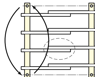
Соединение шин, путем разворота шинодержателя
